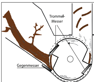
Duplex-Messertrommel
