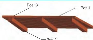
Pos. 1 - Stegbohlen Pos. 2 - Unterkonstruktion aus Vierkantprofilen, schräg angeordnet, einseitig überstehend Pos. 3 - Verschraubung mittels Edelstahl-Senkkschrauben
