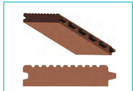
Version 2 - Mit Nut und Feder
