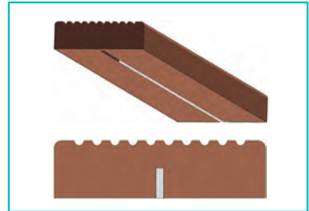
Version 2 - Mit Nut und Feder
