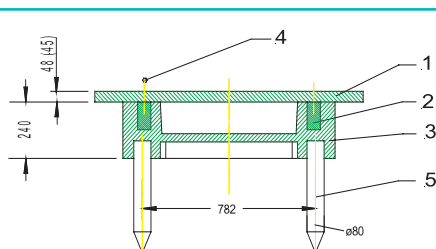
Pos. 1 - Strandwegbretter / Stegbohlen Pos. 2 - Bohlen 6,0x12,0x280 cm - siehe S. 25. Pos. 3 - Traverse Pos. 4 - Abdeckkappen & Schrauben Pos. 5 - Rundpfosten mit Spitze - siehe S. 10.
