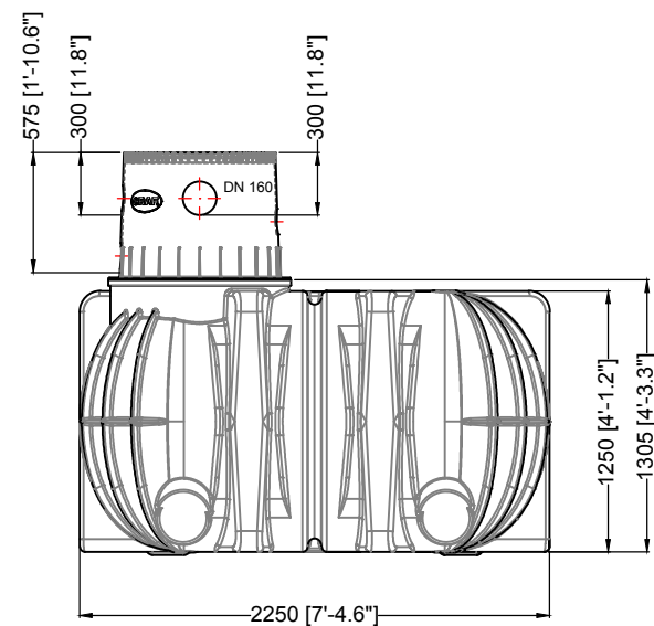
Ansicht A / View A
