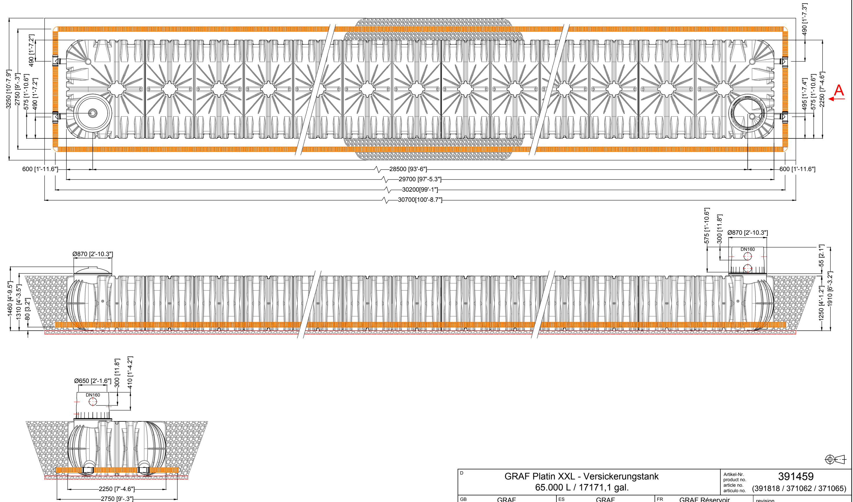
Ansicht A / View A
