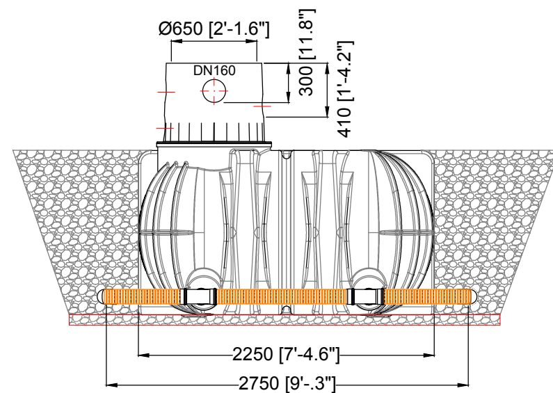
Ansicht A / View A
