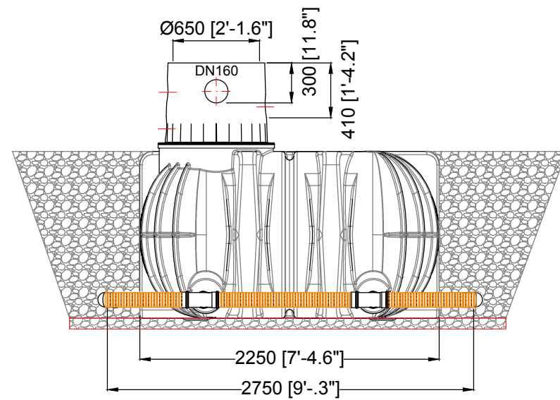
Ansicht A / View A
