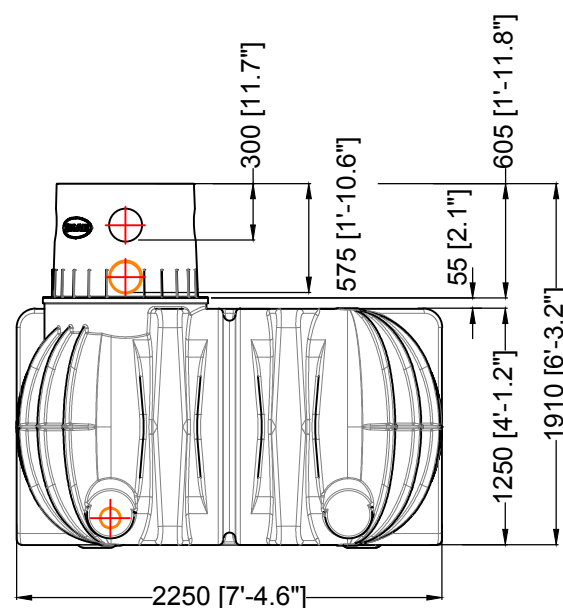
Ansicht A / view A
