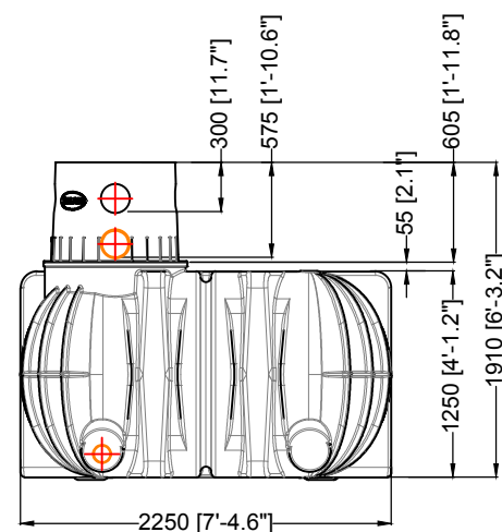
Ansicht / view A
