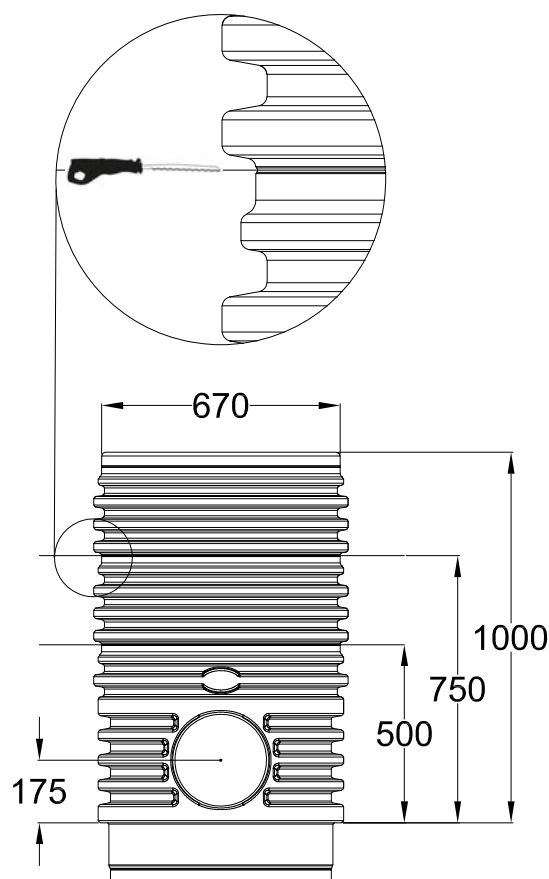
Pieza intermedia VS 1000 DN 600 371015/ 371016
