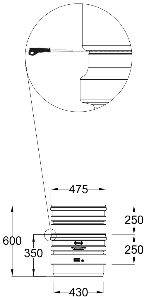
Rallonge pour regard DN 400 330341
